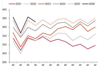
图表 18：中国电解铝产量（单位：万吨）
